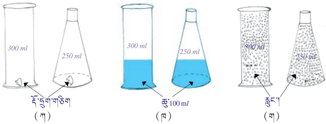
དཔེ་རིས་3.4 (1) སྲ་གཟུགས་ཐམས་ལ་དབྱིབས་དེས་ཅན་ཞིག་ཡོད། (2) གཤེར་གཟུགས་ཀྱིས་སྒོང་དེའི་དབྱིབས་འཛིན་པ་ཡིན། (3) ལྷང་གཟུགས་ཀྱིས་སྒོང་ཆ་ཡོད་པ་འཛིན་པར་བྱེད་ཅིང་། དེ་དག་ལ་དབྱིབས་དེས་ཅན་ཞིག་མེད།
