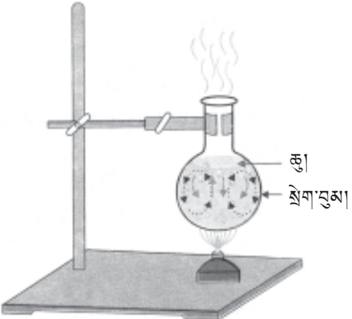
དཔེ་རིས་༡༠་༡༠ ཚོད་ལྟར་འདིས་དྲོད་ཀྱི་འཁོར་བརྒྱུད་བརྒྱུན་ཡོད།
