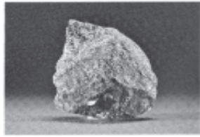
ཟངས་སེར་དོ། (chalcopurite)
