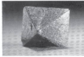
ཟངས་དམར་དོ། (Copper)
