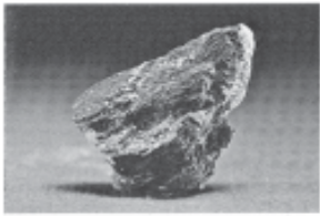
ཟངས་སླུའི་དོ། (Bornite)
