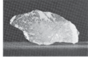
དངུལ་དོ་དཀར་པོ། (Silver)
