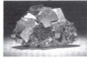
སླ་ཟེའི་དོ། (Pyrite)
