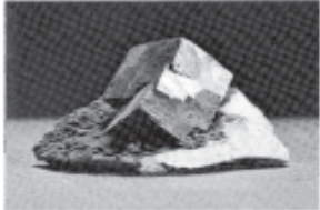
ཞ་ཉེའི་དོ། (Galena)
