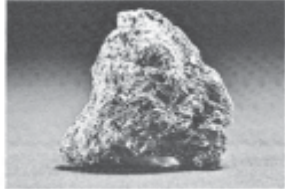
གསེར་དོ། (Gold)
