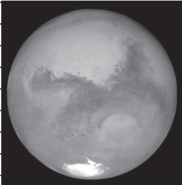
དཔེ་རིས་༡་༥ སའི་གོ་ལ་ནས་མཐོང་བའི་མིག་དམར།
