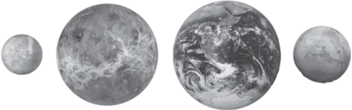
དཔེ་རིས་༡.༡ ལྟེ ལྗེ་སྐར་ལྷག་པ་དང་པ་སངས། སའི་གོ་ལ། མིག་དམར་བཅས་ཀྱི་ཆེ་ཆུང་གནས་སྐབས་རགས་པ།
