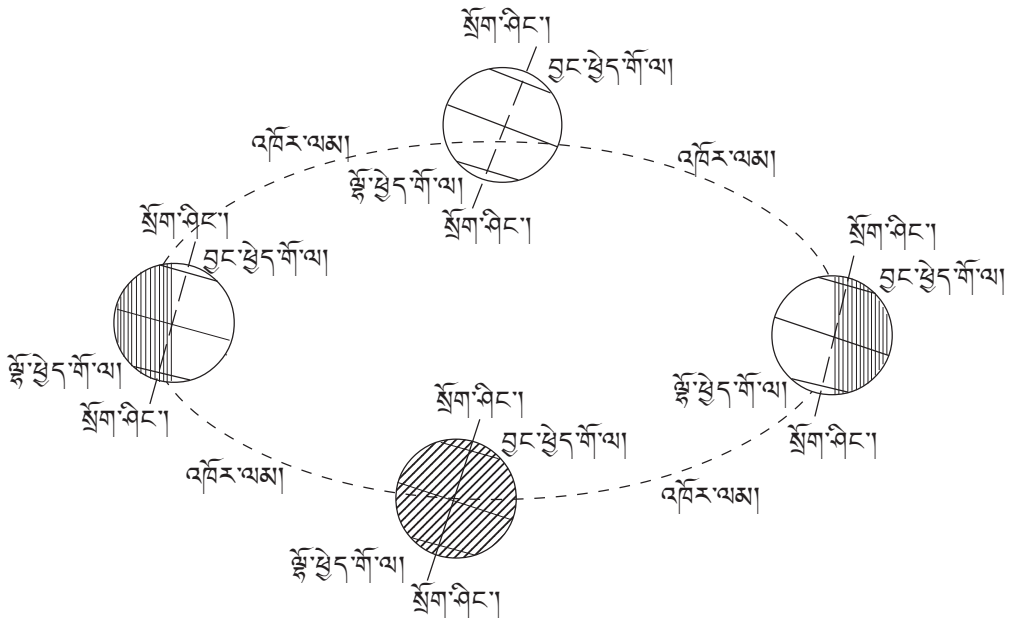
དཔེ་རིས་༡་༥ སའི་གོ་ལས་རང་གི་འཁོར་ལམ་བརྒྱུད་ཉི་མར་གཞན་སྐྱོར་བྱེད་སྐབས་དེའི་གནས་སྤངས་ཀྱི་ཆ་ནས་དང་། སའི་གོ་ལའི་སློབ་ཤིང་ལོ་ནས་རང་འཁོར་བྱེད་སྐབས་ཀྱི་ཆ་ནས་ནམ་དུས་འགྲུར་བ་བྱུང་ཚུལ།
