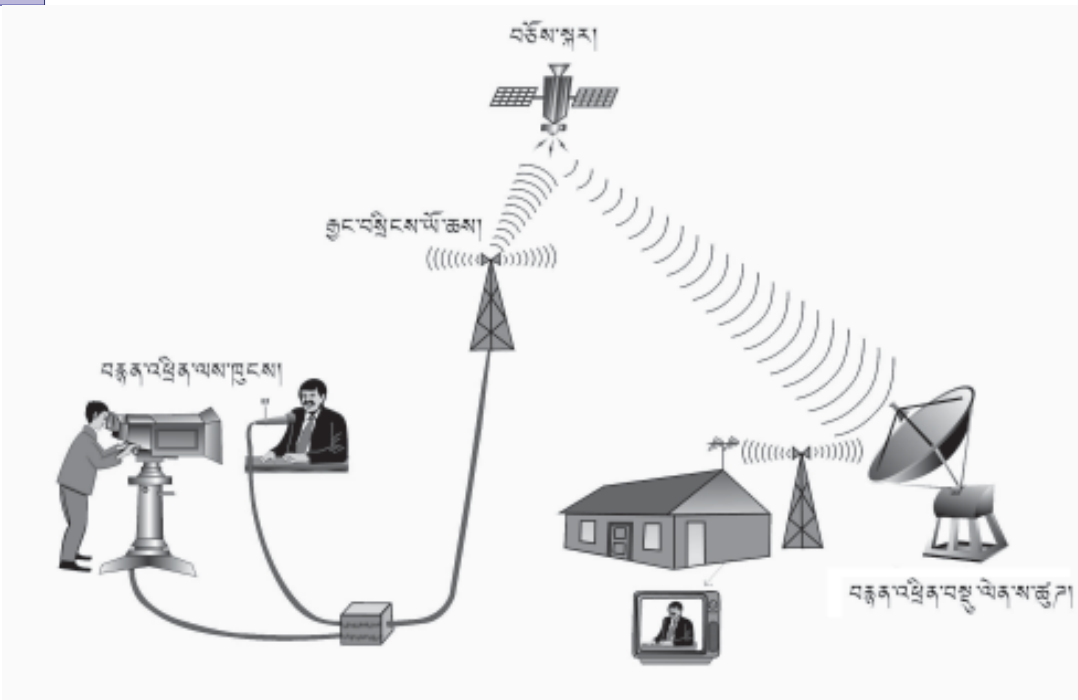
དཔེ་རིས་༡༡༩ བཅོས་མའི་འཁོར་སྐར་བརྒྱན་བརྒྱུ་ལེན་མཚན་བྱང་བསྐྱངས་ཤུད་ཚུལ་གསལ་སྟོན་ཐུབ་པའི་དཔེ་རིས།
