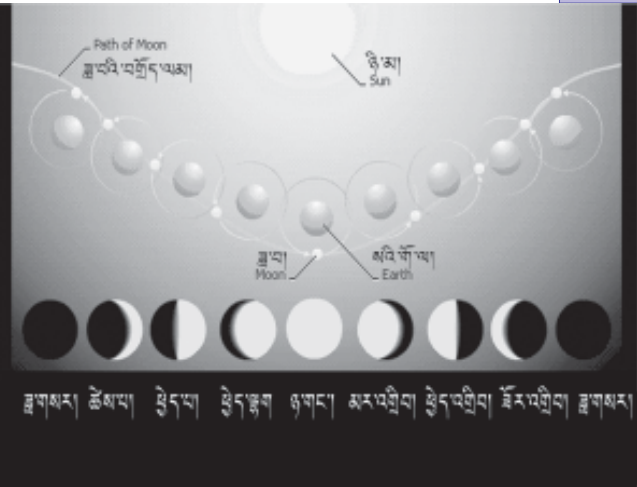
དཔེ་རིས་ ༡་༦ ཀྱི་ ཟླ་བས་སའི་གོ་ལར་རང་གི་འཁོར་ལམ་བརྒྱད་འཁོར་བ་བྱེད་བྱེད་སྐབས་ཀྱི་གནས་སྣང་ས་མི་འདྲ་བ་ཁག་
