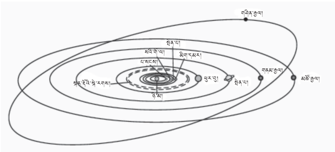
དཔེ་རིས་༡.༡༡ ཉི་མའི་ཁྲིམ་རྒྱུད་ཀྱི་རྒྱ་སྐར་གྱི་ནམ་པ་གཞིགས་བཤེར་བཞུད་པ།
